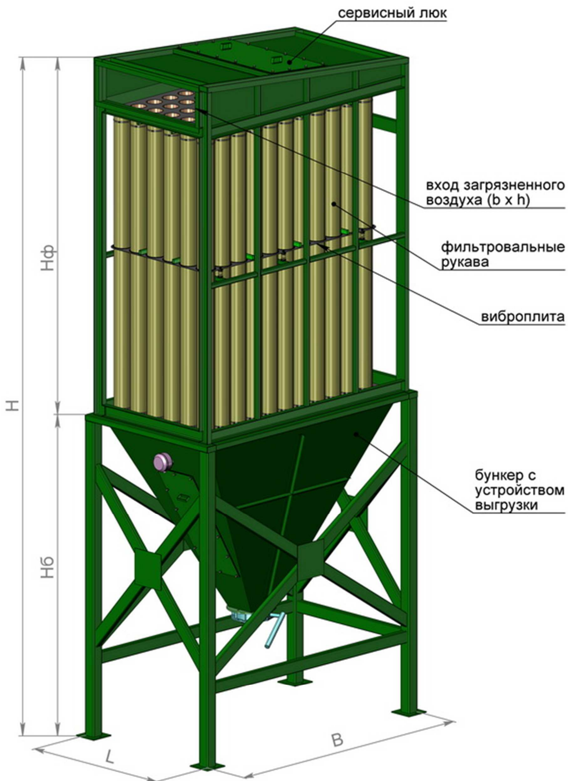
РФУ10 Фильтр рукавный с вибровстряхиванием в бескорпусном исполнении
