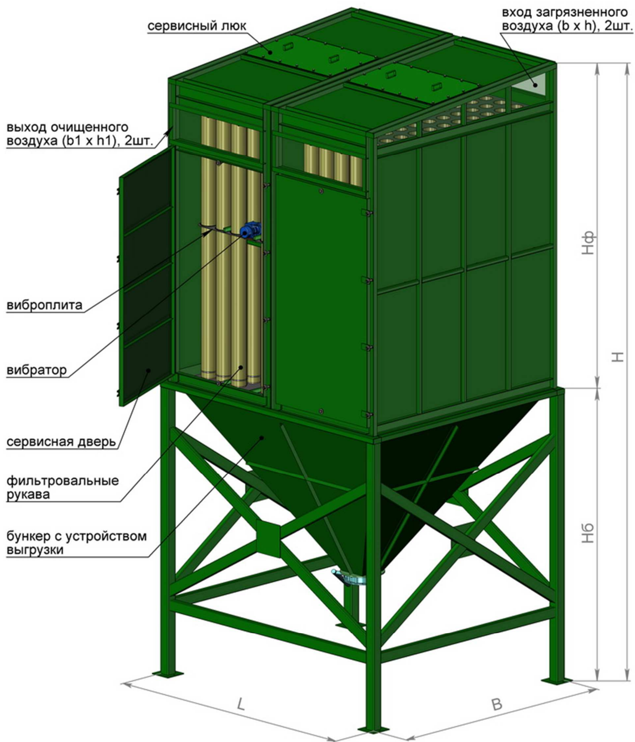
РФУ10x2 Фильтр рукавный двухсекционный с вибровстряхиванием
