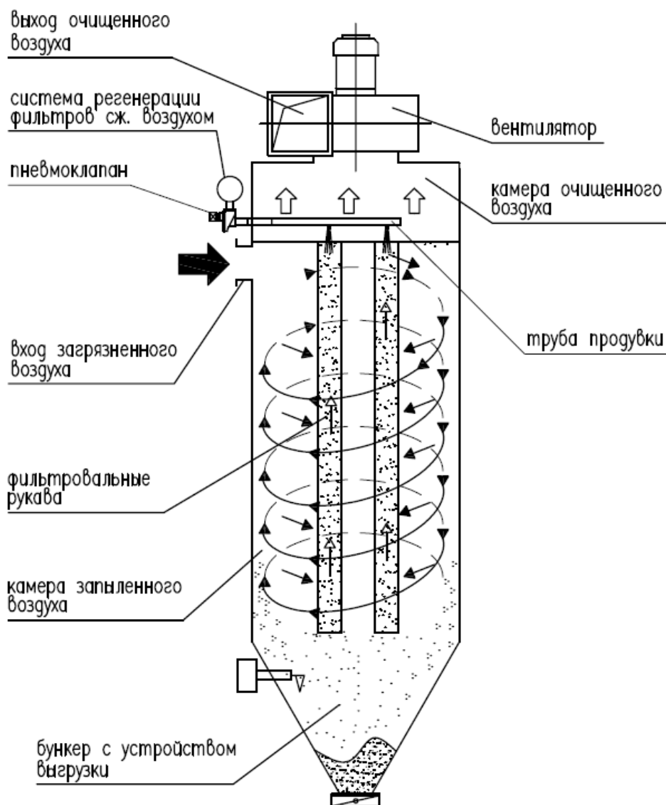
Принципиальная схема фильтровентиляционного агрегата с импульсной продувкой и циклонным входом
