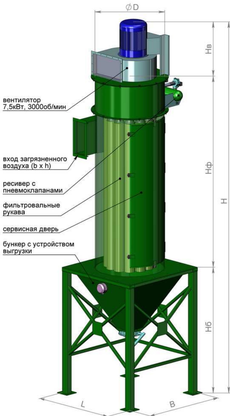
РЦИЭ-ВЕНТ9, РЦИЭ-ВЕНТ18 Фильтровентиляционный агрегат с импульсной продувкой с циклонным входом
