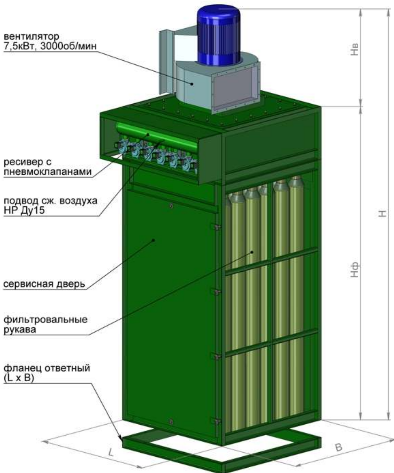
СРФ4-ВЕНТС, СРФ8-ВЕНТС Фильтровентиляционный агрегат с импульсной продувкой в силосном исполнении
