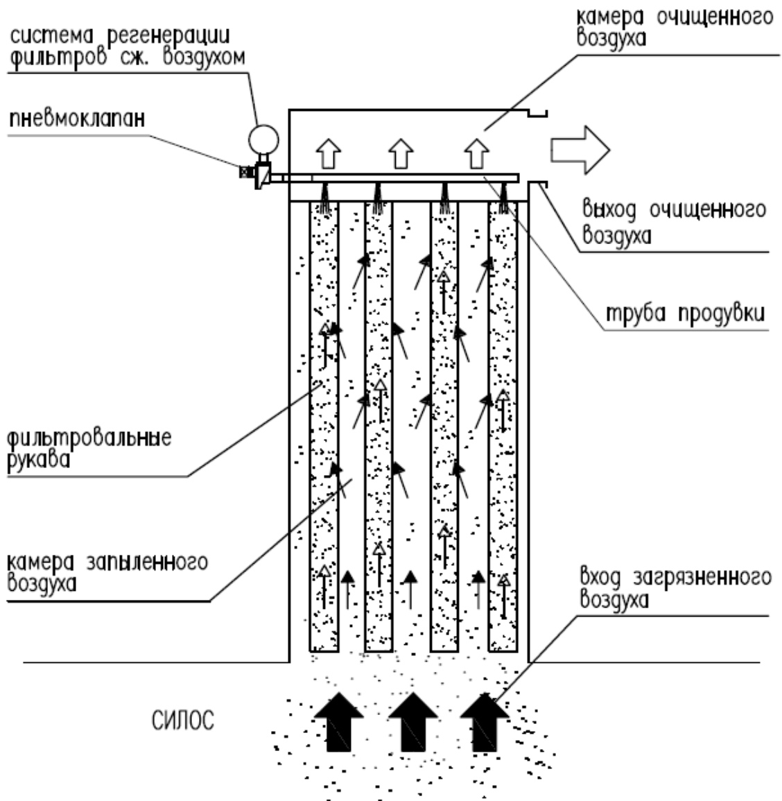
Принципиальная схема рукавного фильтра с импульсной продувкой в силосном исполнении
