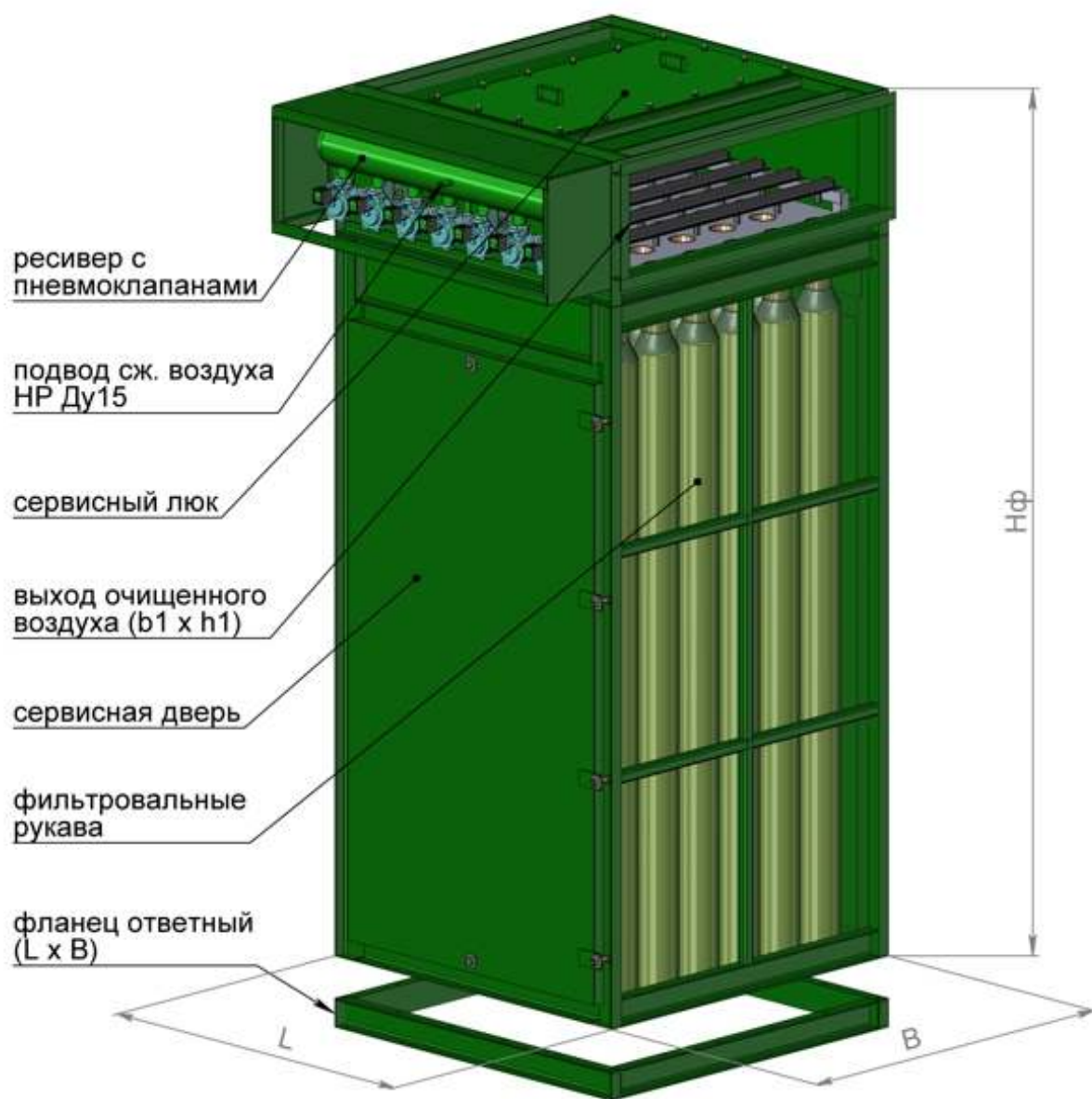
СРФ4С, СРФ8С Фильтр рукавный с импульсной продувкой в силосном исполнении
