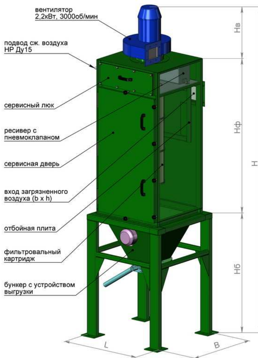
СРФ1К-ВЕНТ Фильтровентиляционный агрегат с импульсной продувкой на базе картриджного фильтра
