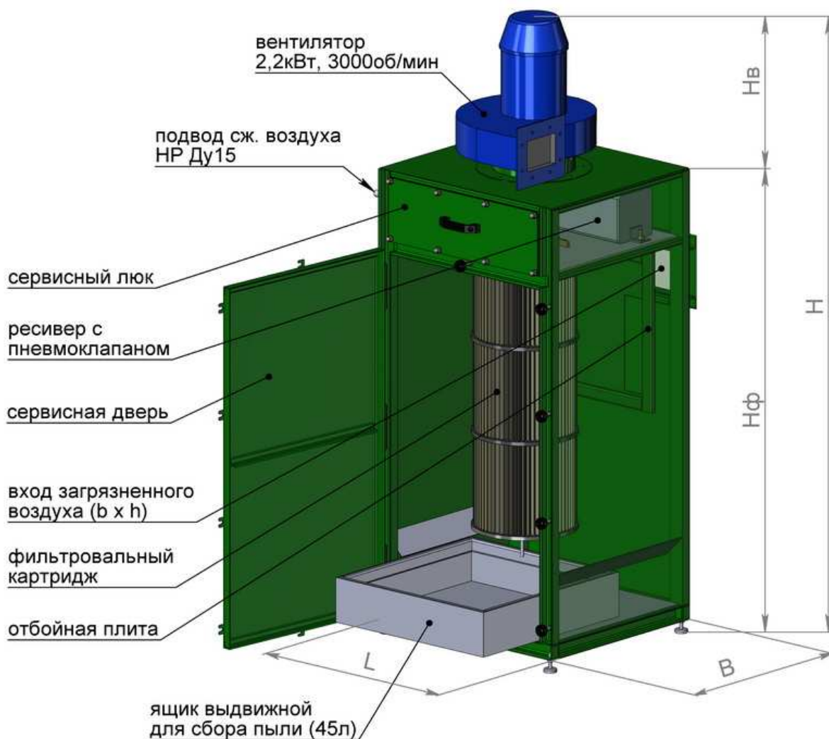
СРФ1КБ-ВЕНТ Фильтровентиляционный агрегат с импульсной продувкой с выдвижным ящиком для сбора пыли
