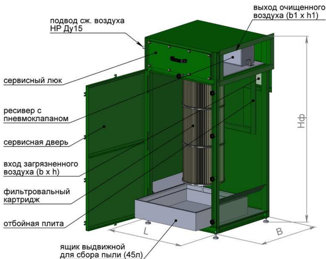
СРФ1КБ Фильтр картриджный с импульсной продувкой с выдвижным ящиком для сбора пыли
