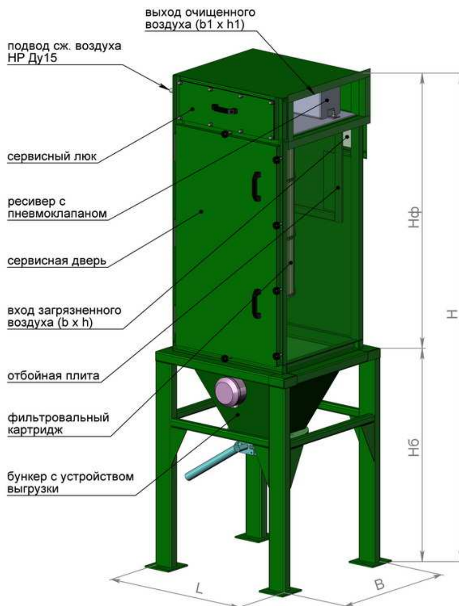
СРФ1К Фильтр картриджный с импульсной продувкой
