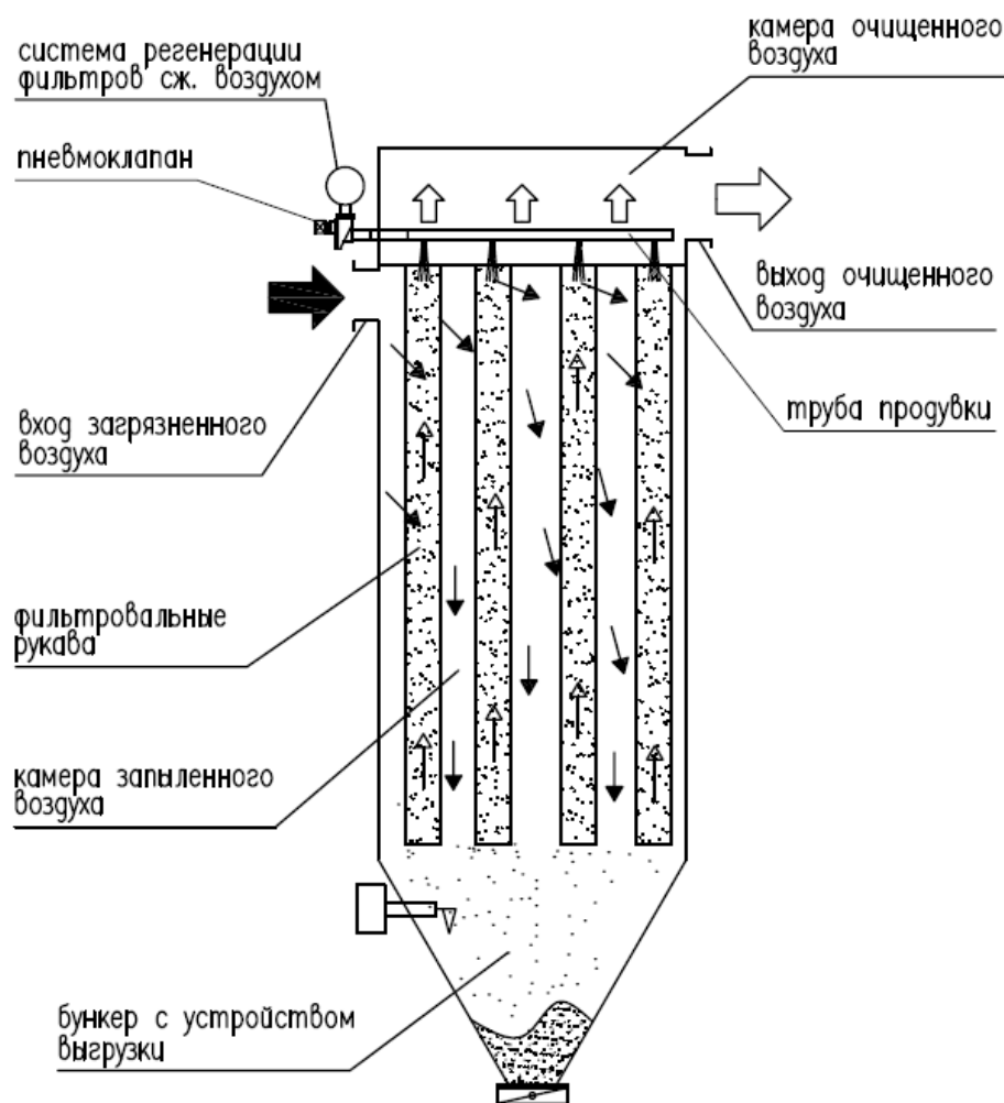
Принципиальная схема рукавного фильтра с импульсной продувкой
