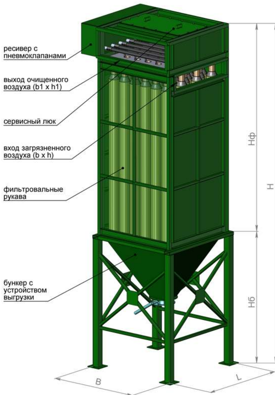
СРФ4, СРФ8 Фильтр рукавный с импульсной продувкой
