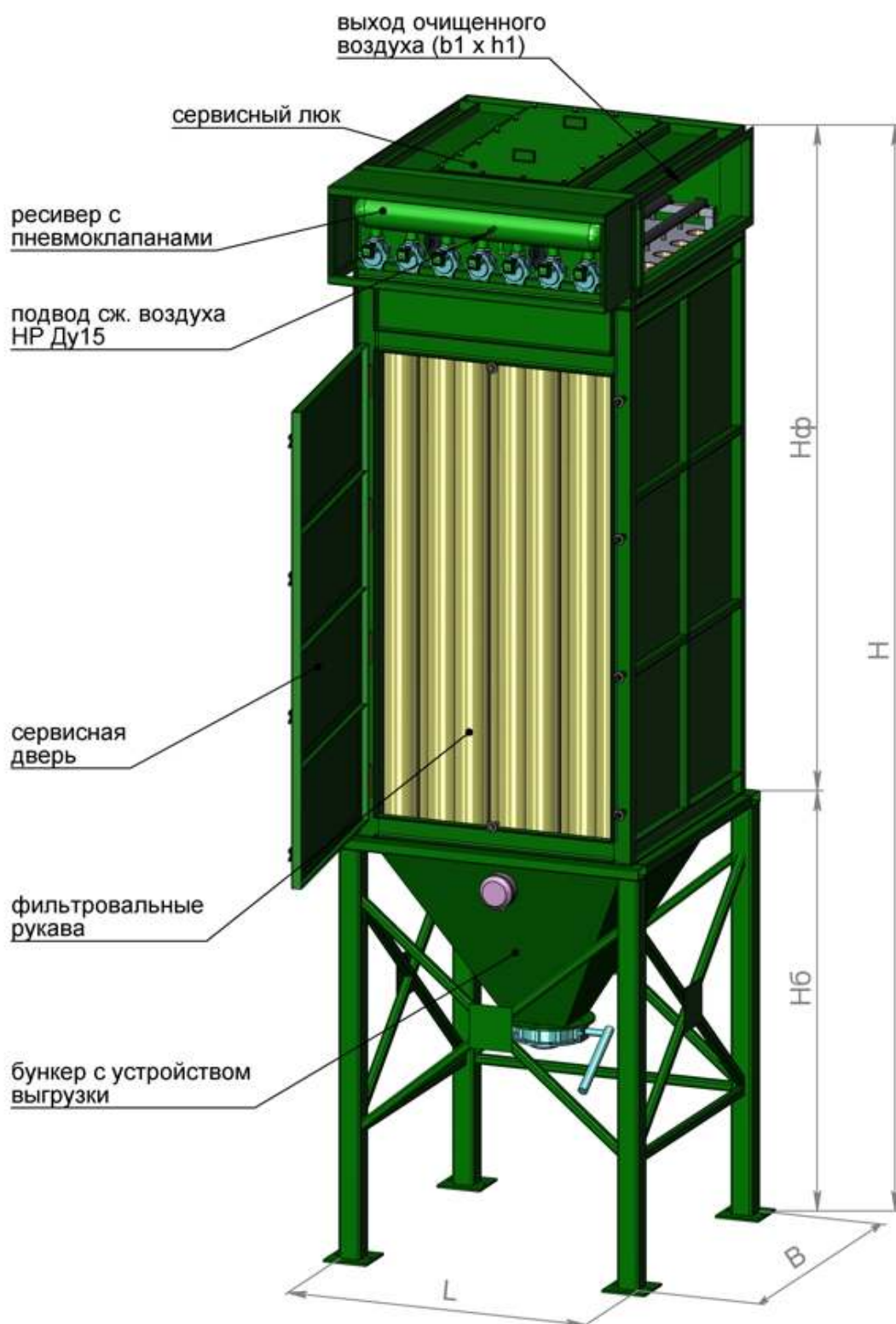
СРФ4, СРФ8 Фильтр рукавный с импульсной продувкой
