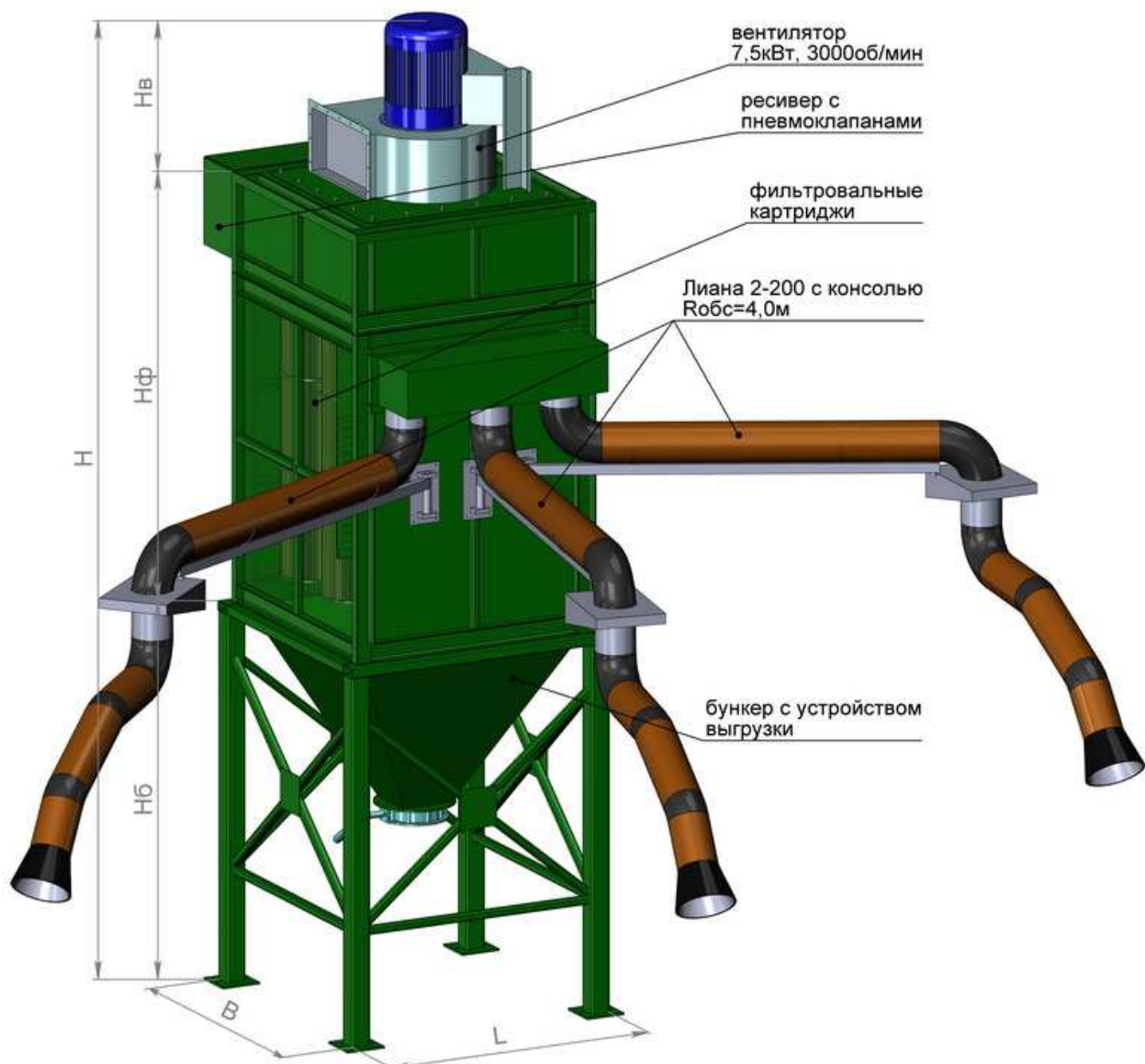
СРФ8К-ВЕНТ-ЛИАНА Фильтровентиляционный агрегат с импульсной продувкой и тремя местными вытяжными устройствами (МВУ)
